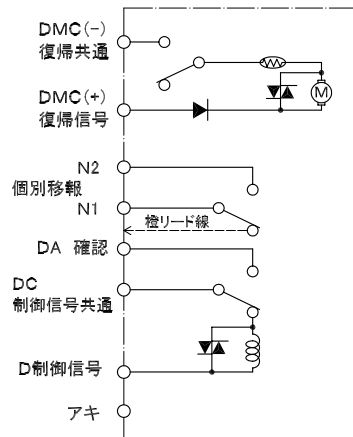
内部回路図 (作動前)
