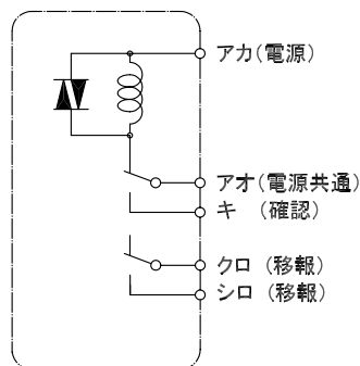
内部回路図(作動前)
