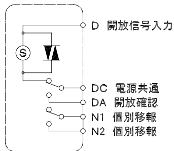
内部回路図(注:待機状態を示す)
