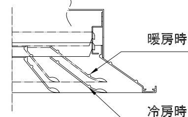
冷房時~暖房時 切替要領図 (S=1/4)
