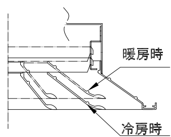
冷房時～暖房時 切替要領図 (S=1/4)
