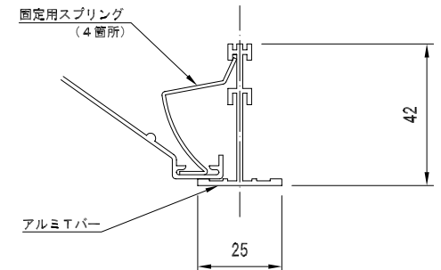
A部詳細 (S = 1 / 2) 水平吹出のみ
