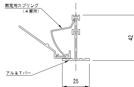
A部詳細 (S = 1 / 2) 水平吹出のみ
